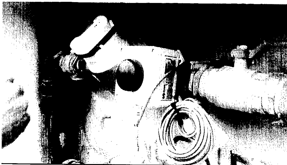
Figura 10. Instalação de um datalogger associado a contador de água
